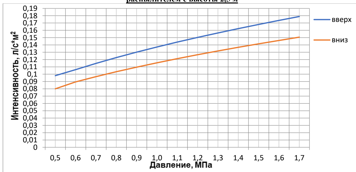
График зависимости интенсивности орошения от давления на площади 9 м2, защищаемой группой распылителей (два и более) с высоты 2,5 м
